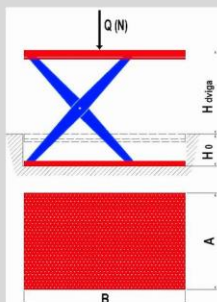
Glavne karakteristike dvižnih miz.
